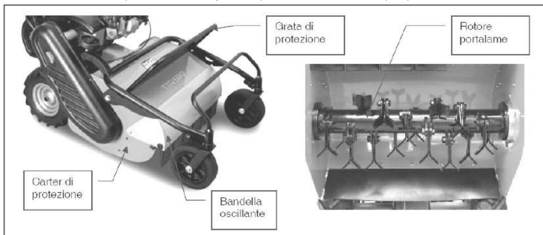
Fig. 3 Apparato di trinciatura
