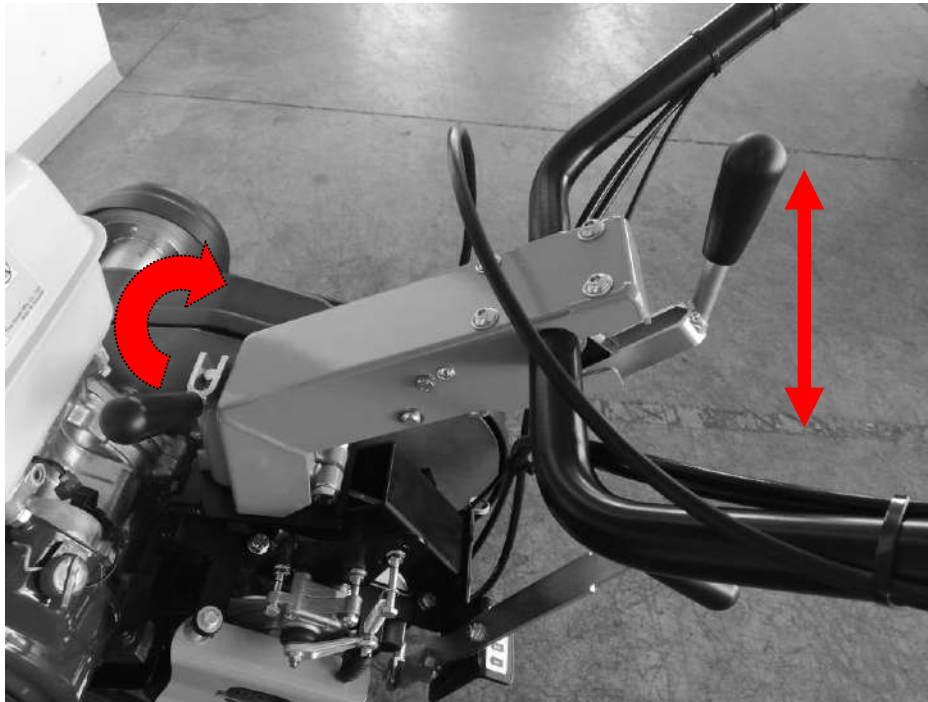
Fig. 122 Regulación del manillar
